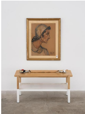
AES-PoPRS16
