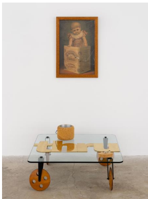
AES-PoPRS8
